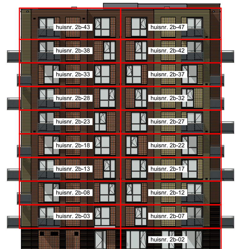
achtergevel hoogbouw
