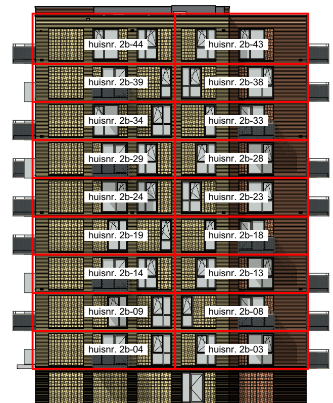
rechter zijgevel hoogbouw
